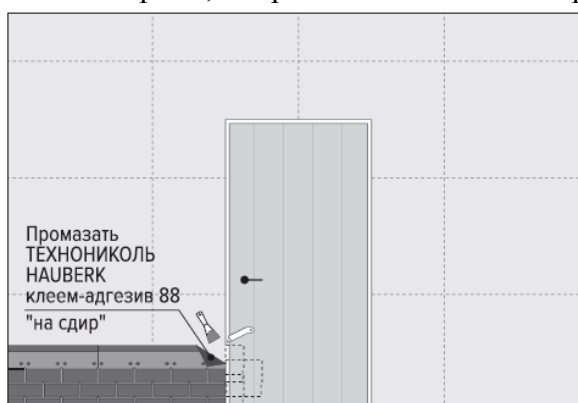
Рис.7.1 Монтаж фасадной плитки вокруг дверных проемов
