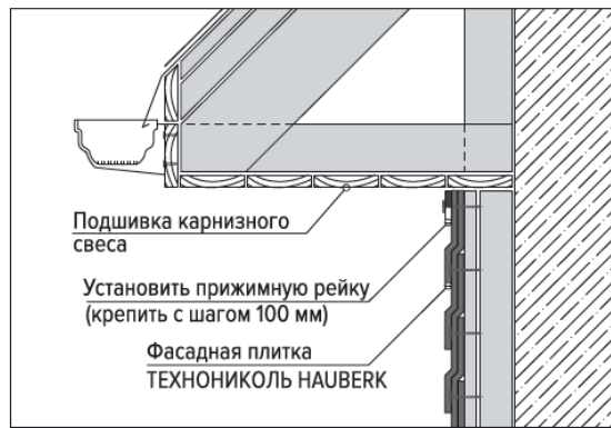
Рис.9.2 Монтаж верхнего ряда под карнизным свесом. Вариант 2
