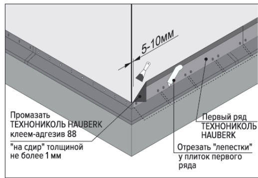
Рис.4.1 Монтаж первого ряда фасадной плитки
