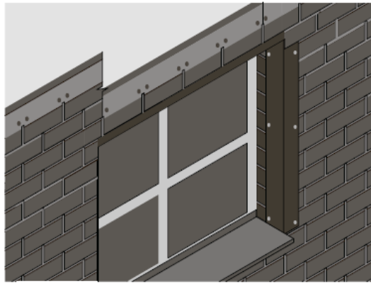
Рис.8.4 Монтаж уголка внешнего сверху проема
