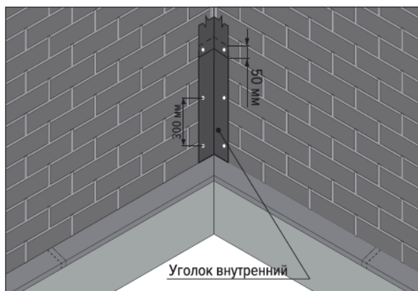
Рис.6.3 Устройство внутренних углов
