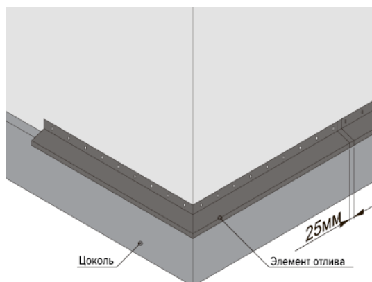
Рис.3.1 Установка цокольного отлива
