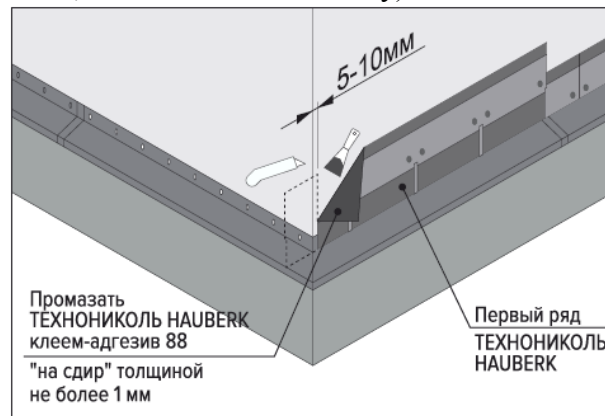
Рис.4.2 Монтаж второго и последующих рядов фасадной плитки
