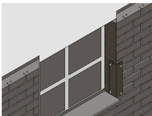
Рис.8.3 Монтаж уголка внешнего сбоку проема
