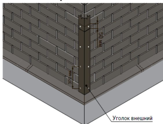
Рис.5.1 Устройство внешних углов
