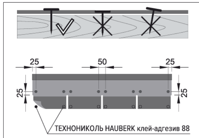
Рис.1.1 Схема крепления фасадной плитки
