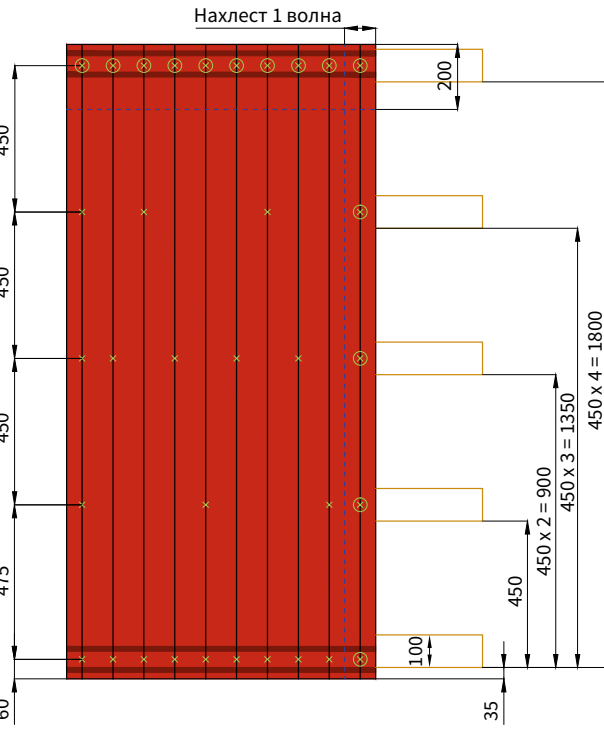
УГОЛ НАКЛОНА КРЫШИ 10- 15°
